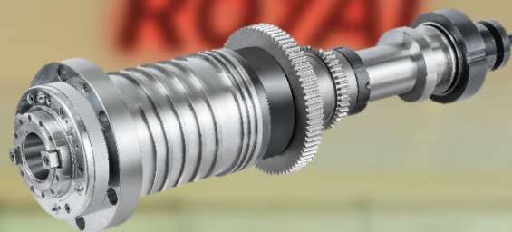
齒輪式主軸
